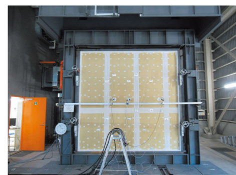
非耐力壁の試験状況
