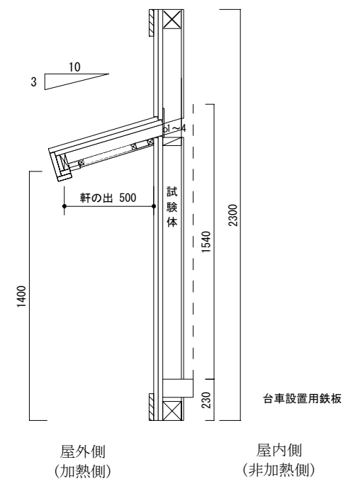
鉛直断面図
