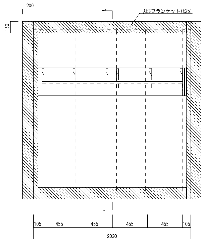
屋外側正面図(加熱側)
