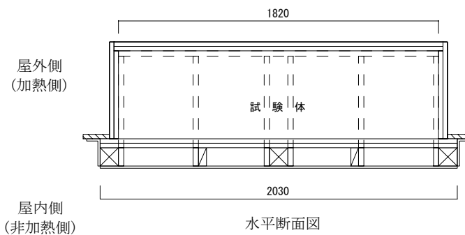
図-＊ 試験体の構造・寸法・温度測定位置(寸法単位: mm)
