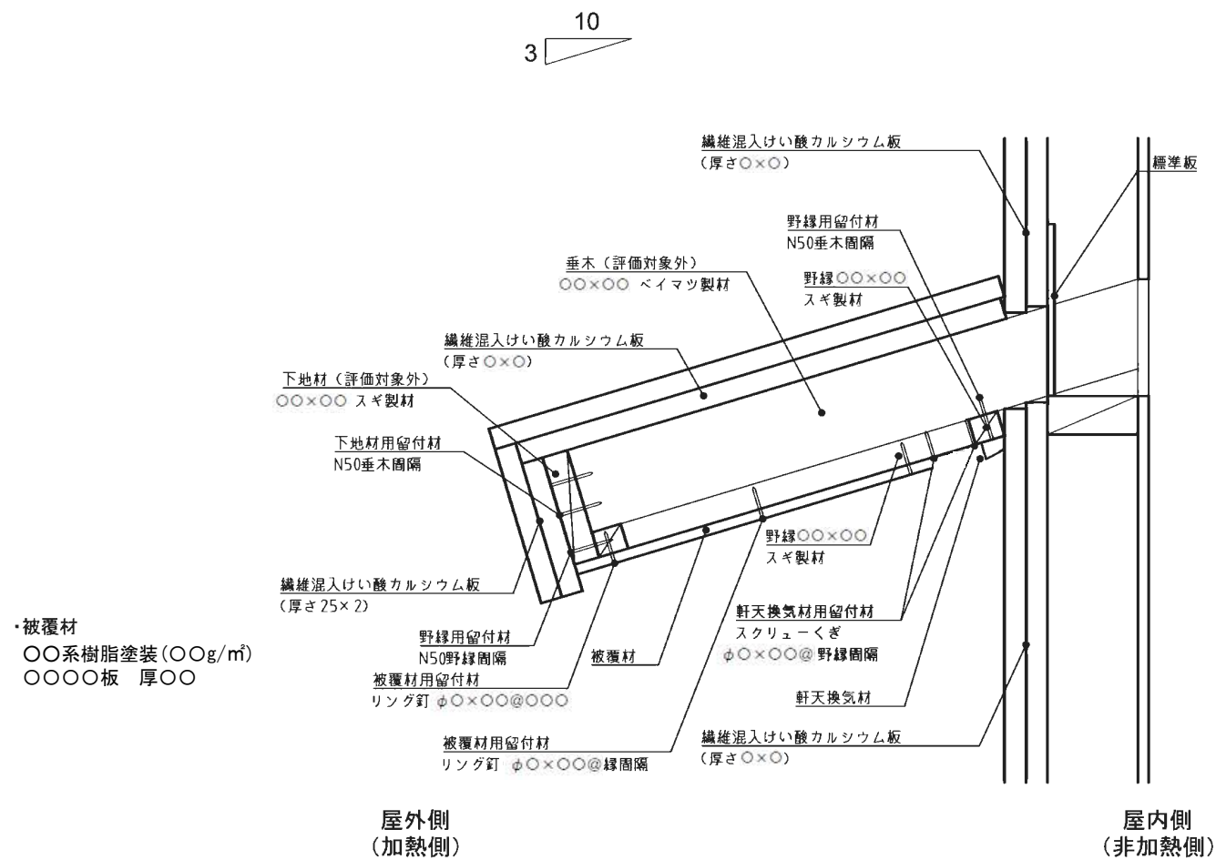
鉛直断面詳細図
