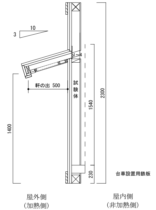
鉛直断面図
