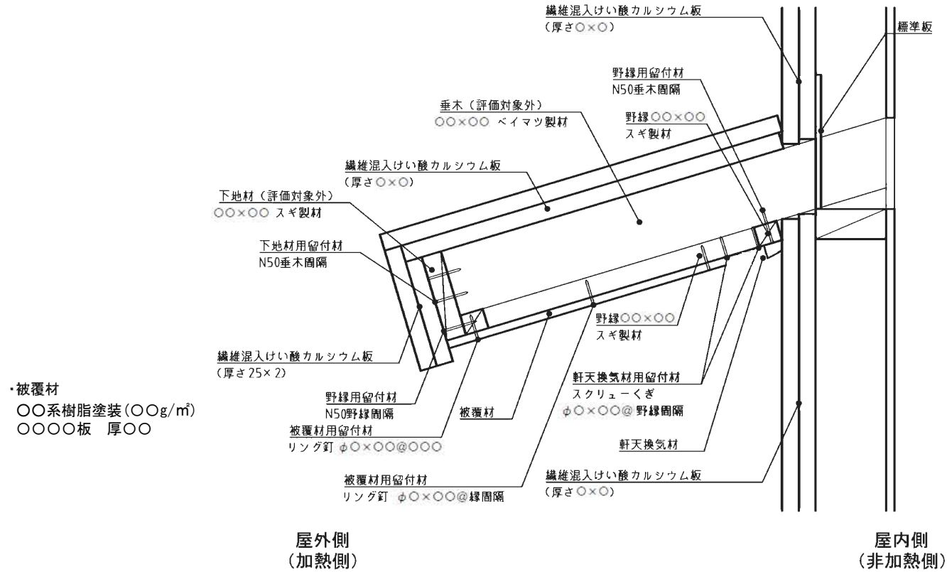
鉛直断面詳細図
